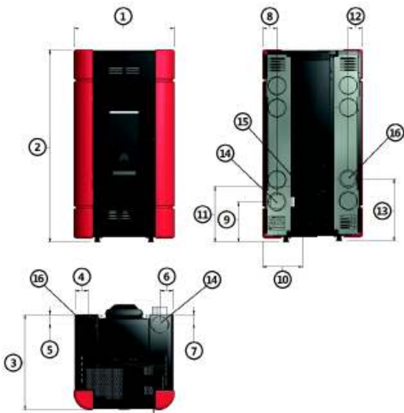
Fig. 13 - Dimensiones generales: Sire Plus
