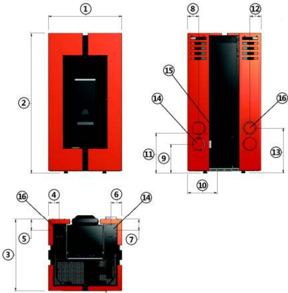
Fig. 14 - Dimensiones generales: Doge Plus
