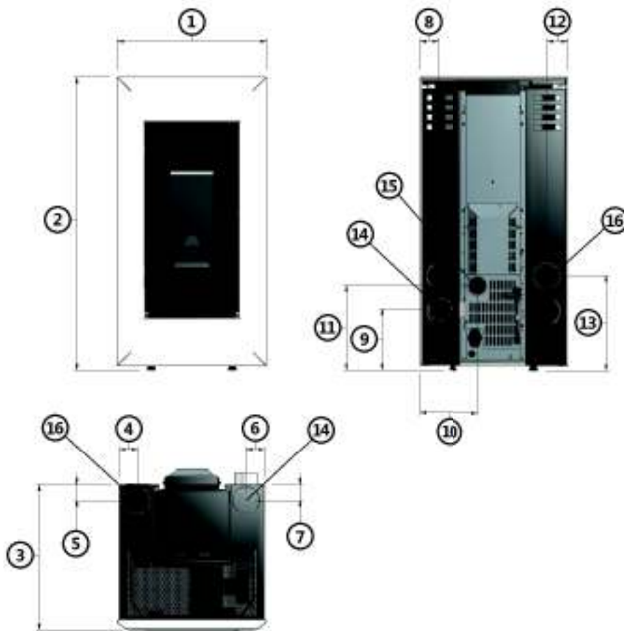
Fig. 12 - Dimensiones generales: Vega
