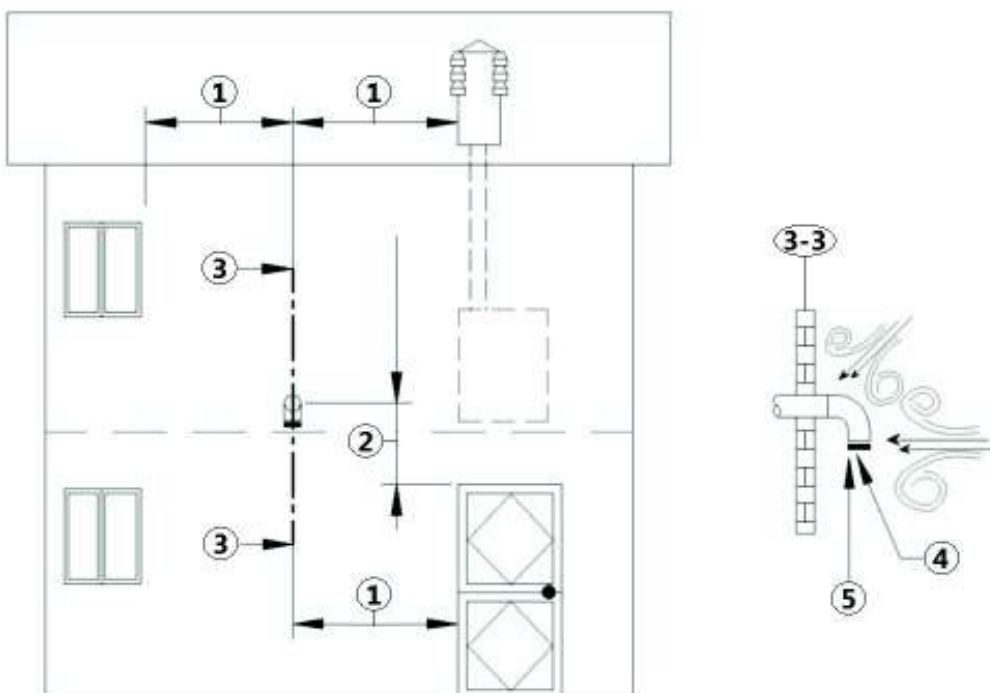
Fig. 8 - Toma de aire en caso de instalación estanca
