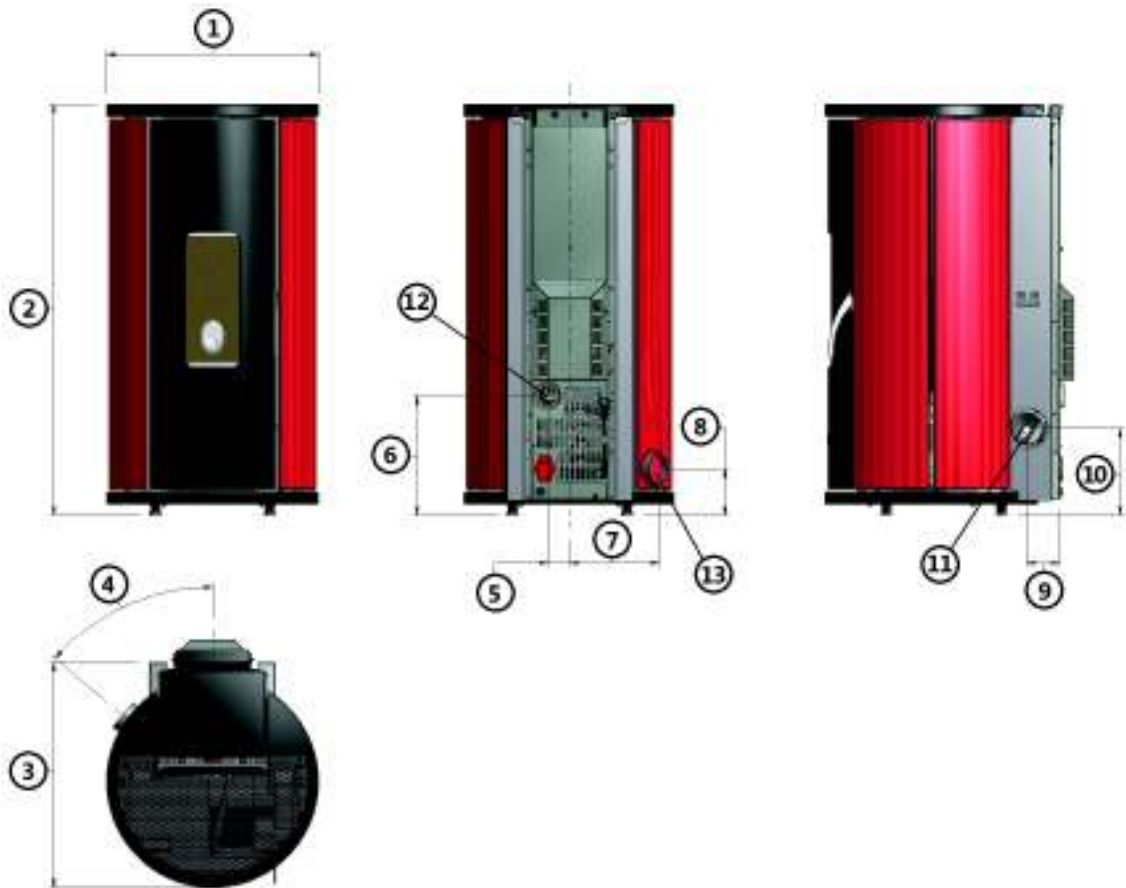
Fig. 15 - Dimensiones generales: Sfera / Sfera Plus
