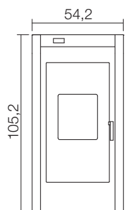
vista fronte stufa
