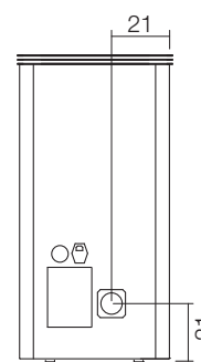
vista retro stufa
