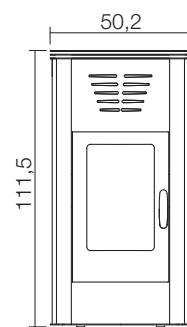
vista fronte stufa
